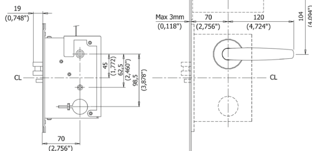
Cerradura de embutir JPN:
