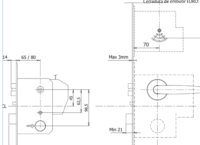
Cerradura de embutir EURO:
