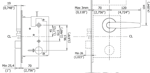
Cerradura de embutir ANSI DA:
