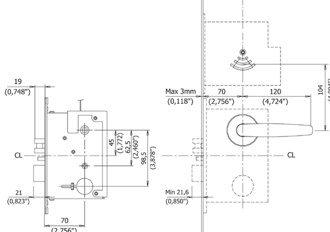
Cerradura de embutir JPN:
