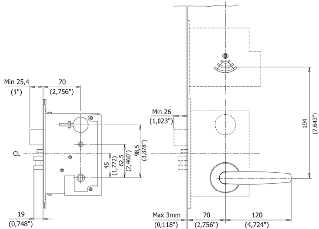
Cerradura de embutir ANSI DA:
